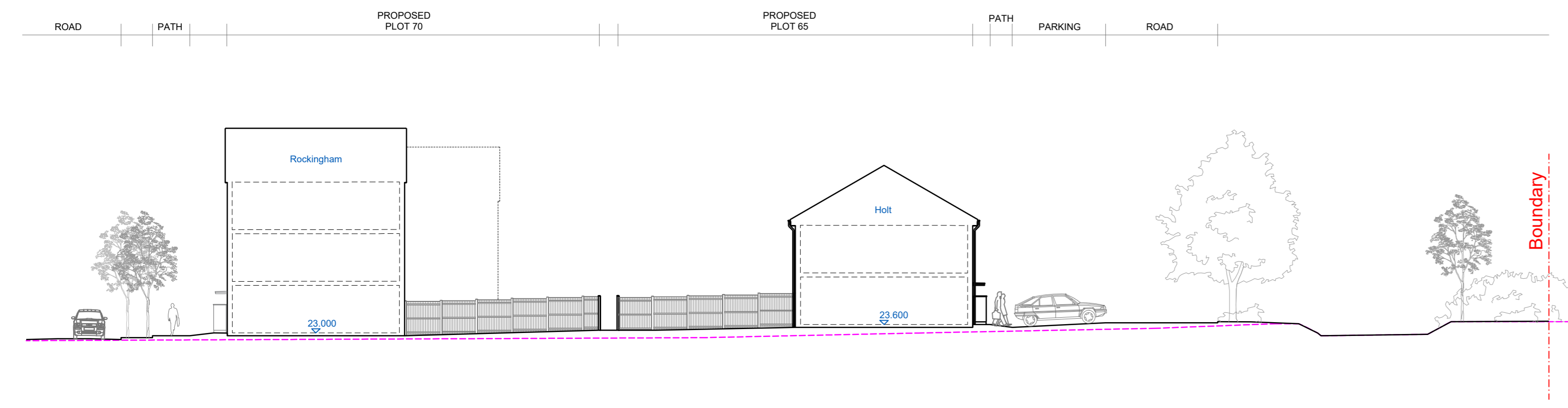
DATUM - 15.00 SECTION C-C
